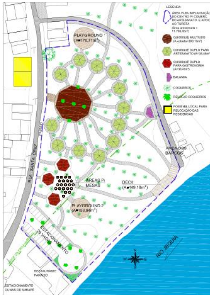
Figura 6 – Implantação do Centro para Comercialização do Artesanato e Apoio ao Turista, localizado no povoado Barra de Jequiá, Jequiá da Praia-AL. Sem escala.
