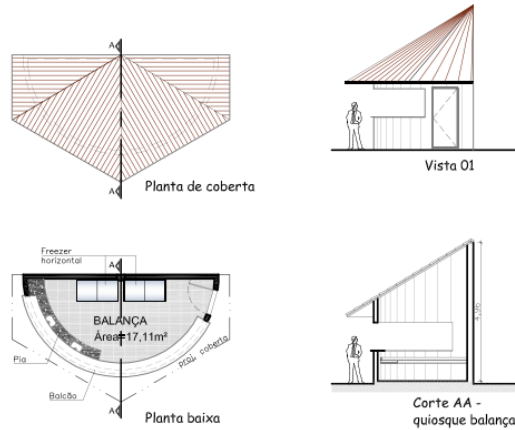
Figura 9 – Quiosque Balança, proposto para o Centro para Comercialização do Artesanato e Apoio ao Turista, localizado no povoado Barra de Jequiá, Jequiá da Praia-AL. Sem escala.
