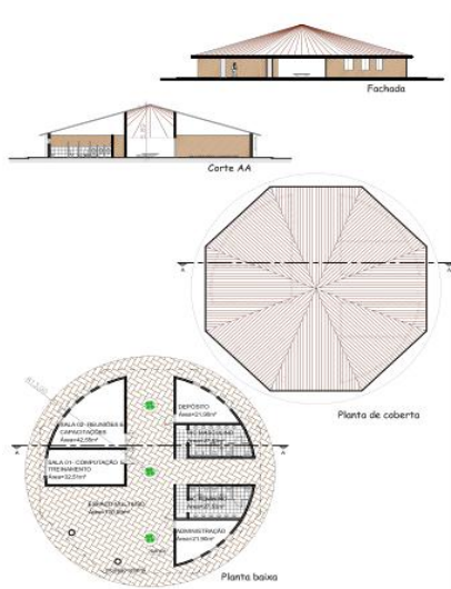
Figura 7 – Quiosque Multiuso, Quiosque Artesanato, propostos para o Centro para Comercialização do Artesanato e Apoio ao Turista, localizado no povoado Barra de Jequiá, Jequiá da Praia-AL. Sem escala.
