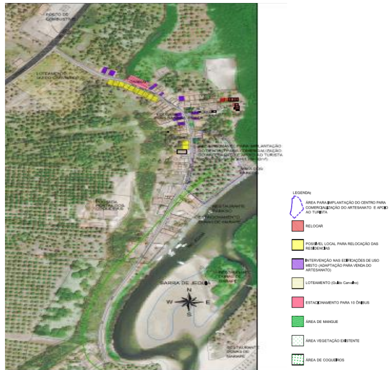
Figura 4 – Implantação geral da proposta de Desenho Urbano para a Barra de Jequiá.
